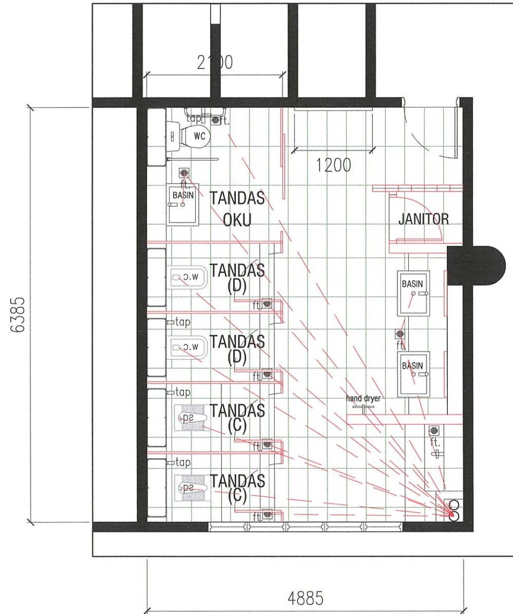
PELAN SANITARI (TANDAS WANITA)
