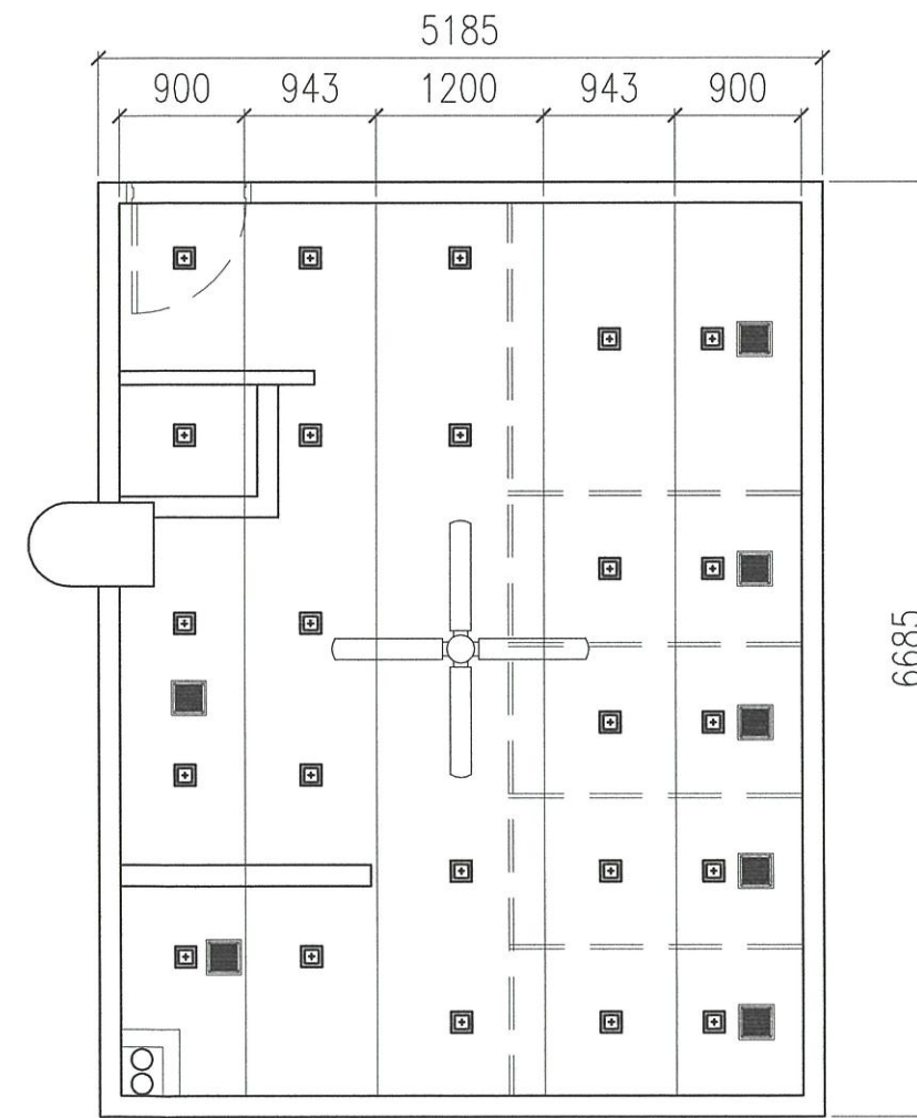
PELAN SILING - TANDAS LELAKI
