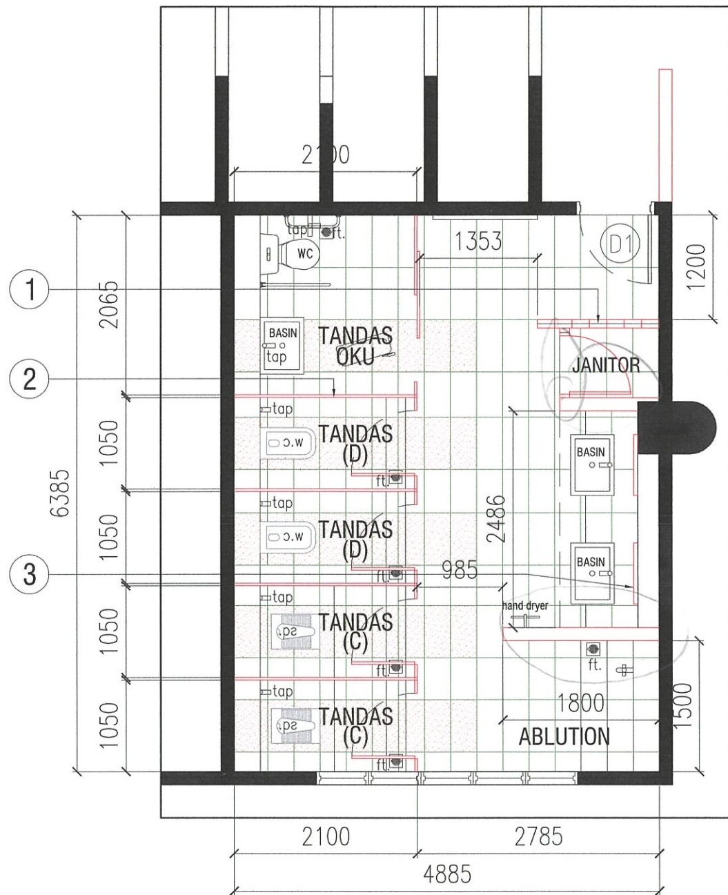
PELAN LANTAI TANDAS WANITA
