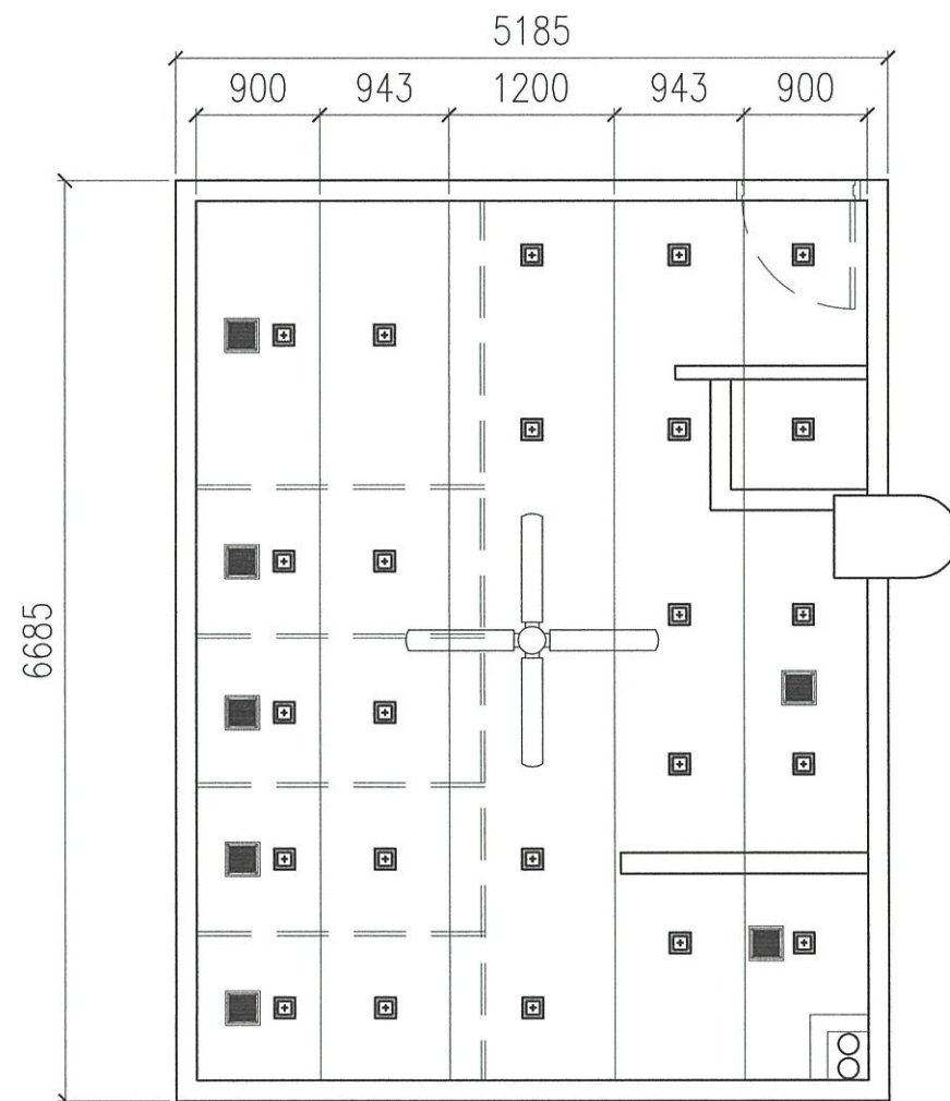
PELAN SILING - TANDAS WANITA
