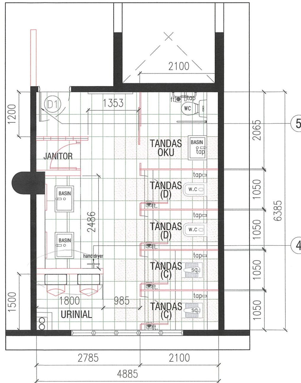
PELAN LANTAI TANDAS LELAKI
