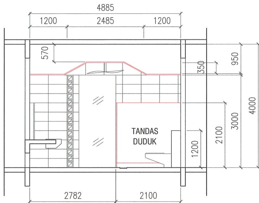
KERATAN A-A
