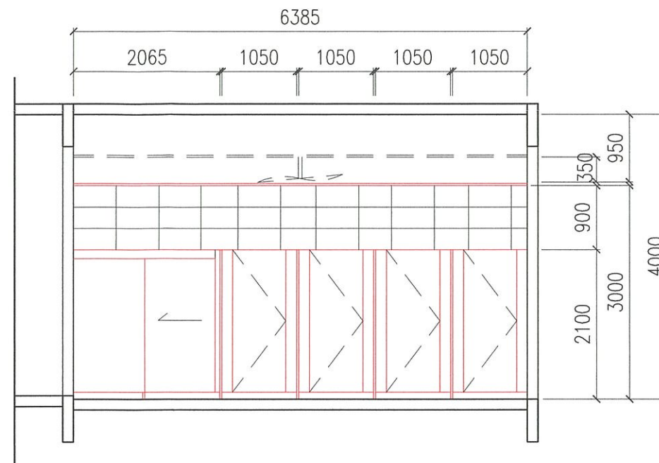
KERATAN B-B
