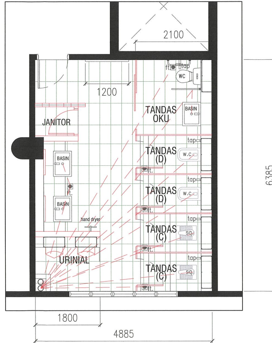
PELAN SANITARI (TANDAS LELAKI)
