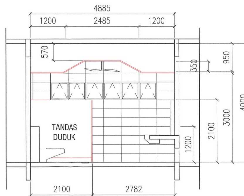
KERATAN D-D
