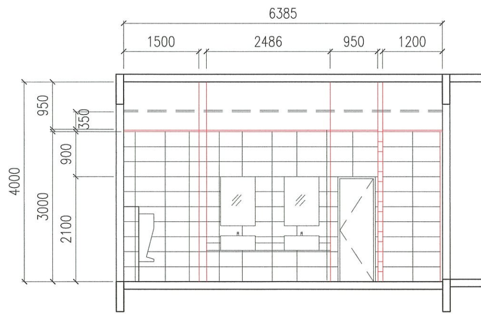
KERATAN C-C
